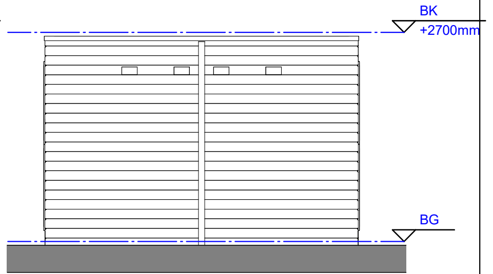
Rechter zijgevel
