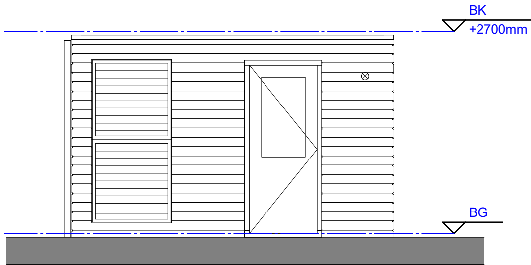
Achtergevel
