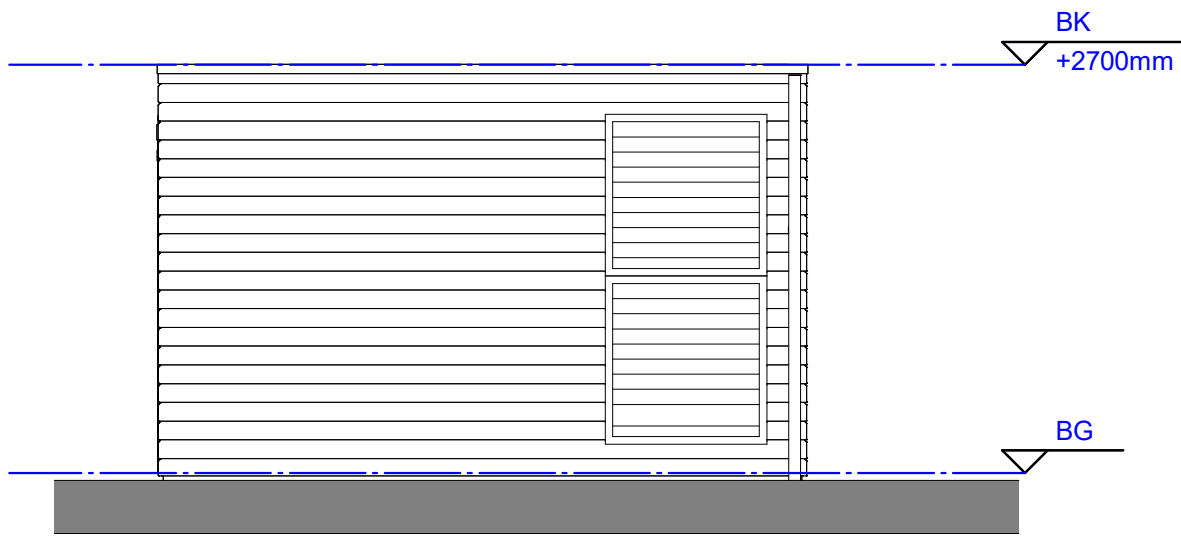
Voorgevel 1 : 50
