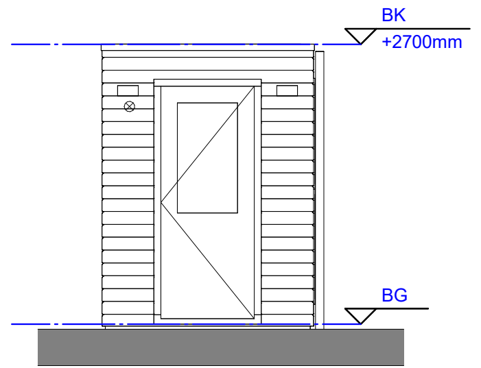
Linker zijgevel 1 : 50
