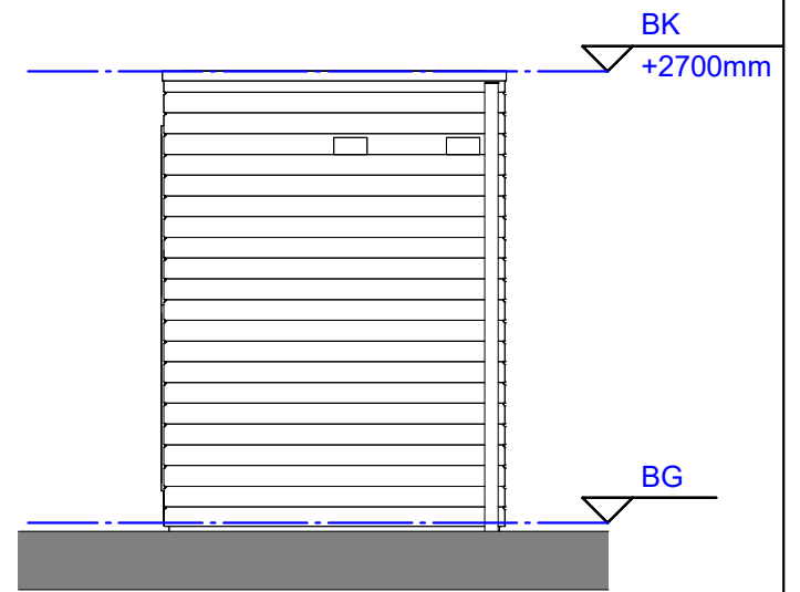
Rechter zijgevel 1 : 50
