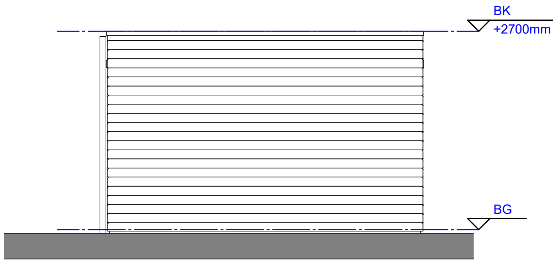
Achtergevel 1 : 50
