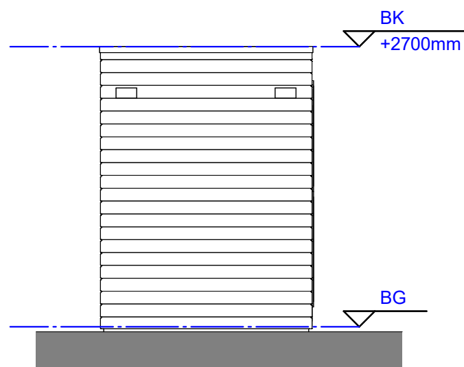
Linker zijgevel
