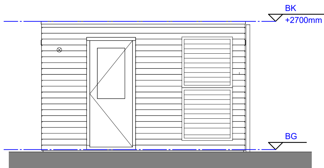
Voorgevel
